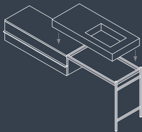
Telaio portasalviette H. 769 a terra L. 776-926 Per piani lavabo integrato H. 120
